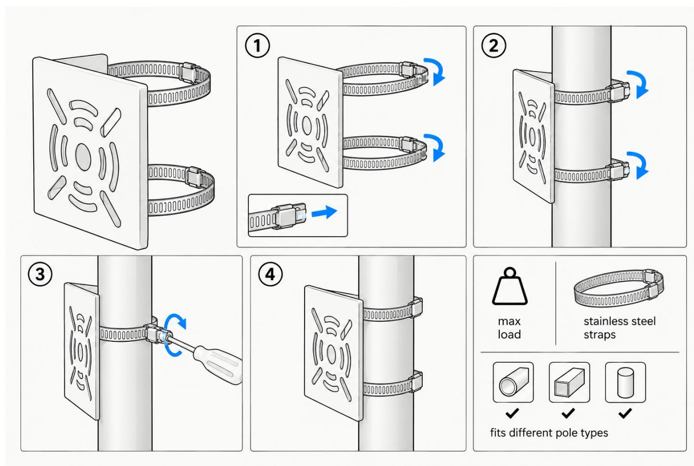
Rys.1. Montaż
